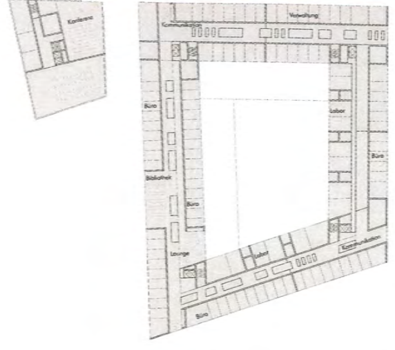
Regelgeschöß ‚Science Tower‘ M 1:500
