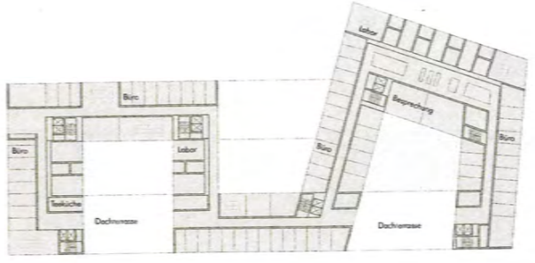
Regelgeschöß Laborgebäude M 1:500
