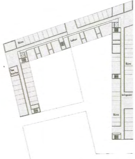
Regelgeschöß ‚Produktion‘ M 1:500
